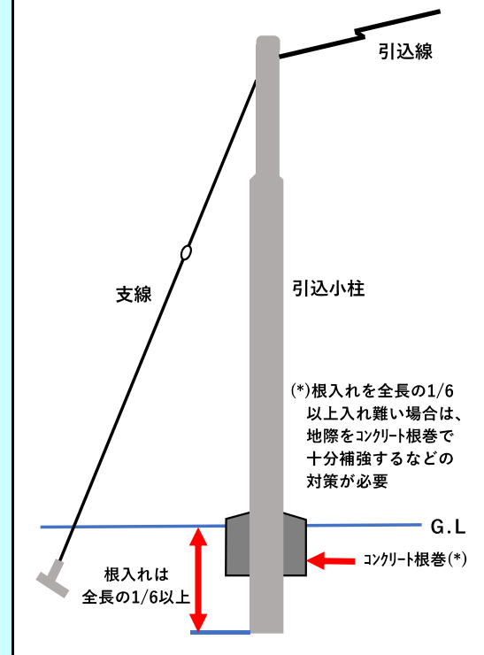
【図2】引込小柱などの施工例 ※ 詳細は、内線規程 資料2-2-3「引込小柱などの標準施工図例」を確認ください
